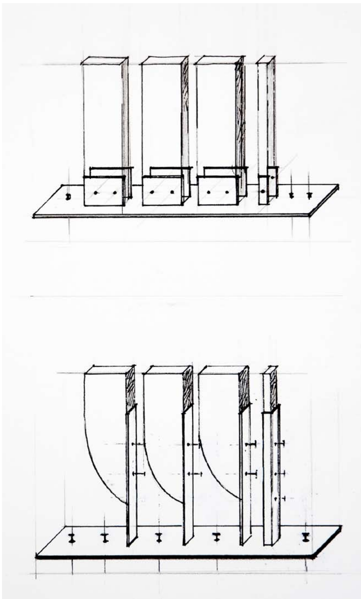
Systèmes de fixations / sol Sabots ou ferrures acier de 5 mm, sablés et peints, visserie.
